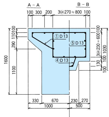
断面図
