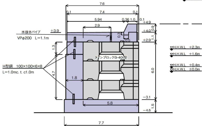
標準断面図
