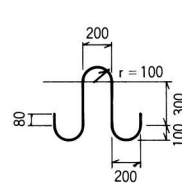
⑩ φ19 × 1710
