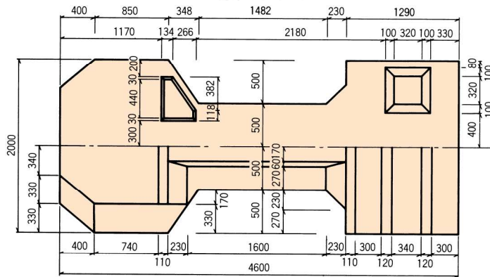
平面図
