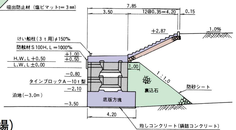
標準断面図
