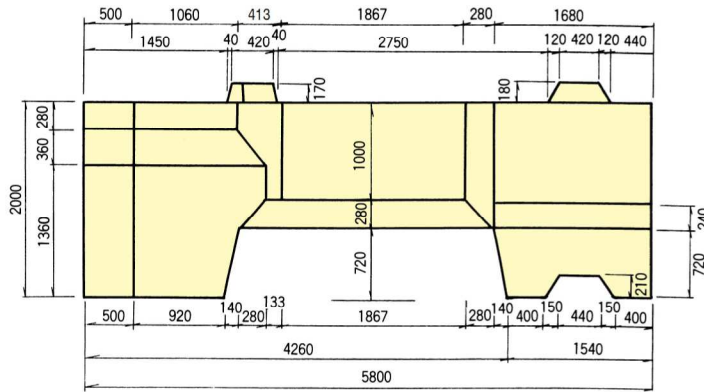
平面図
