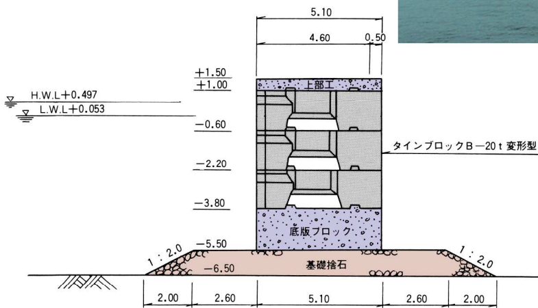
標準断面図
