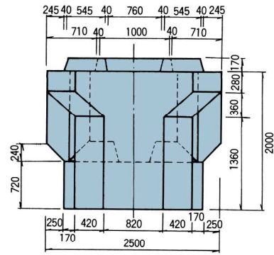
正面図
