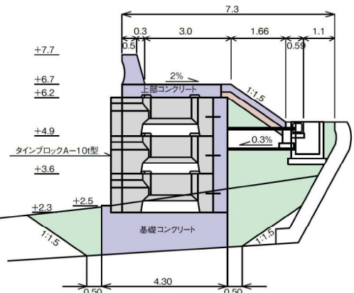
標準断面図
