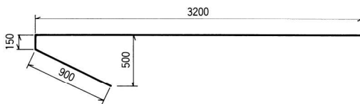
⑨ D16 × 2460
