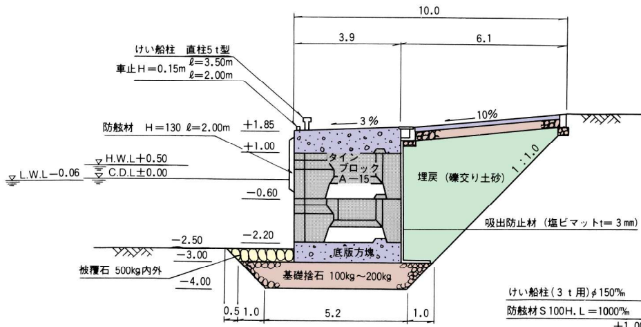
標準断面図
