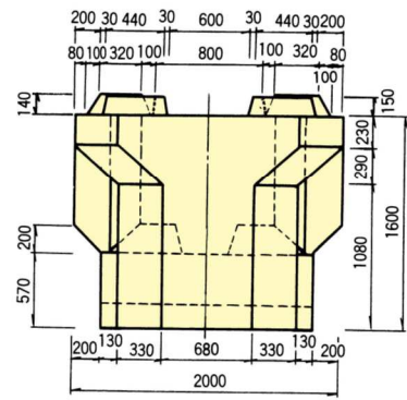
正面図
