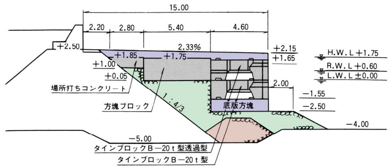
標準断面図
