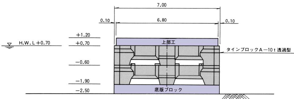
標準断面図
