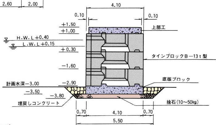
標準断面図
