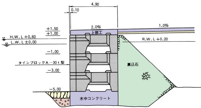
標準断面図
